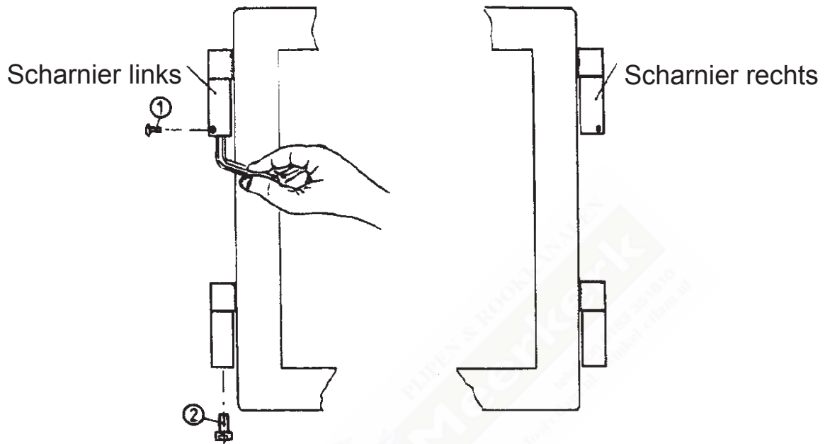
Figuur 4: Scharnieren
